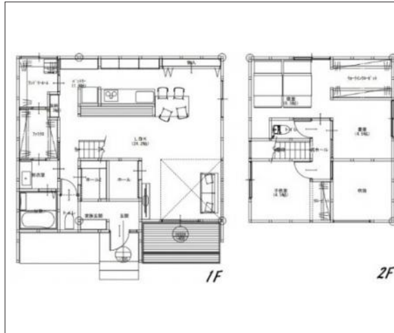
間取り図
